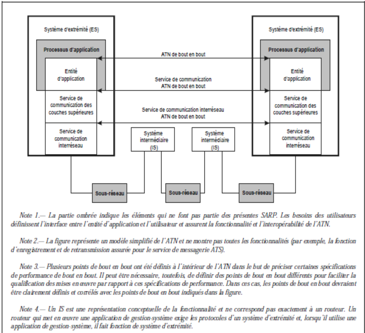
Figure 3-1. Modèle conceptuel de l'ATN
