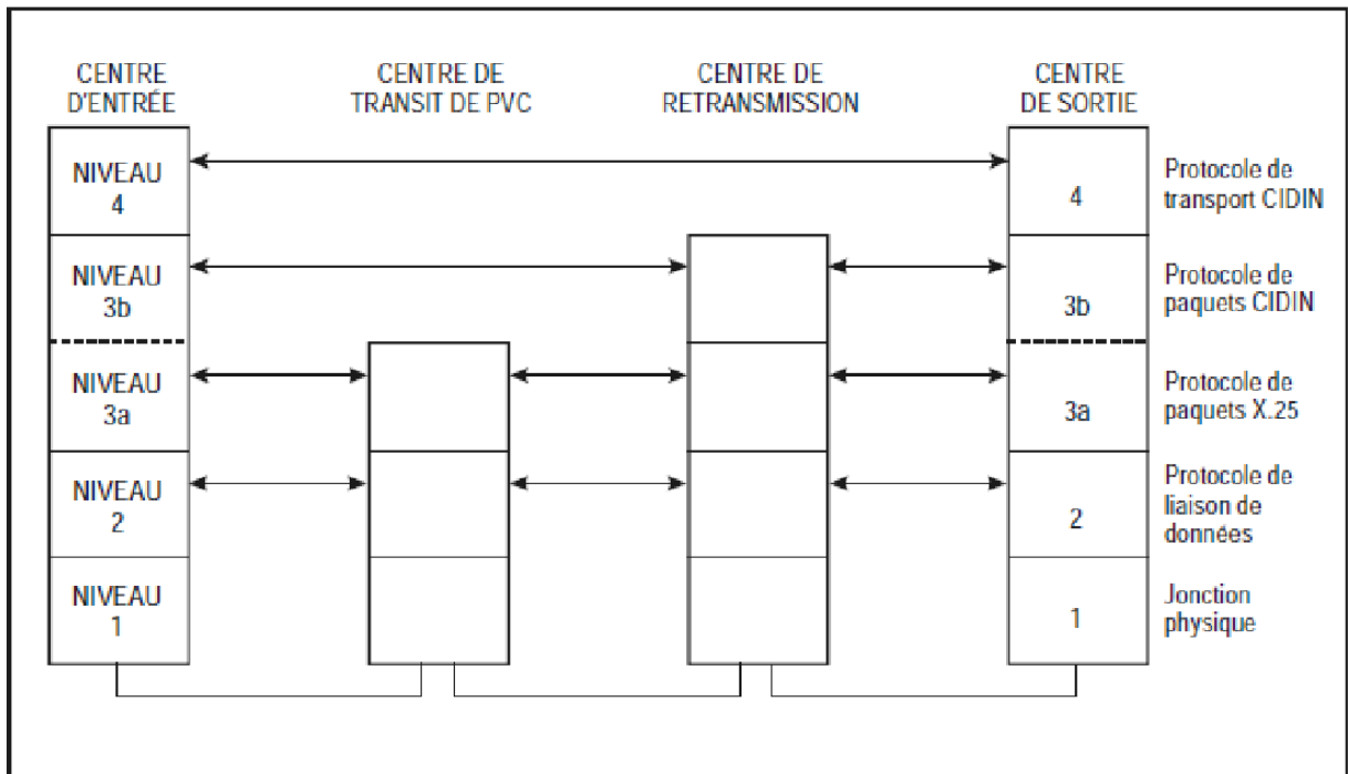
Figure 8-1. Niveaux de protocole CIDIN
