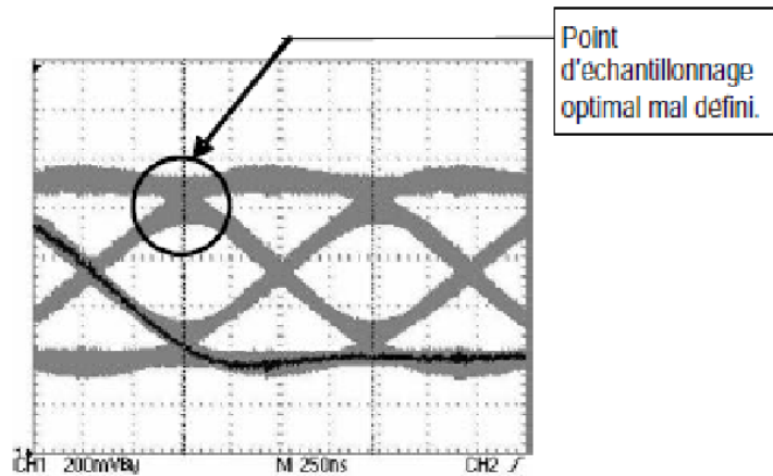
Figure 12-4. Diagramme en œil déformé
