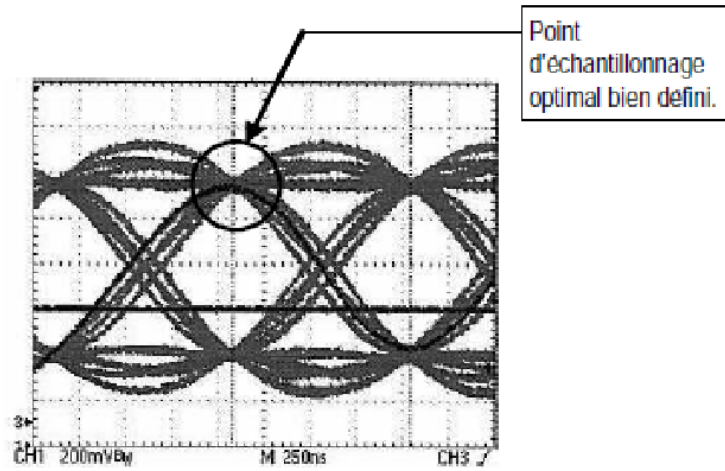
Figure 12-3. Diagramme en œil idéal
